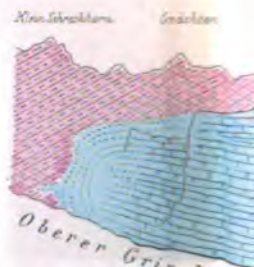
Fig. 9. Halbschematische Ansicht des Mettenbergs.
